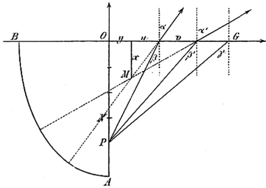
Abb. 5: Das Diagramm zur Entstehung des Hebungspunktes bei Bauer [13]. Die zwei von P ausgehenden Lichtwege treten unter den Winkeln \alpha und \alpha' aus der Grenzfläche aus und kreuzen sich in der rükwärtigen Verlängerung im Bildpunkt M .
